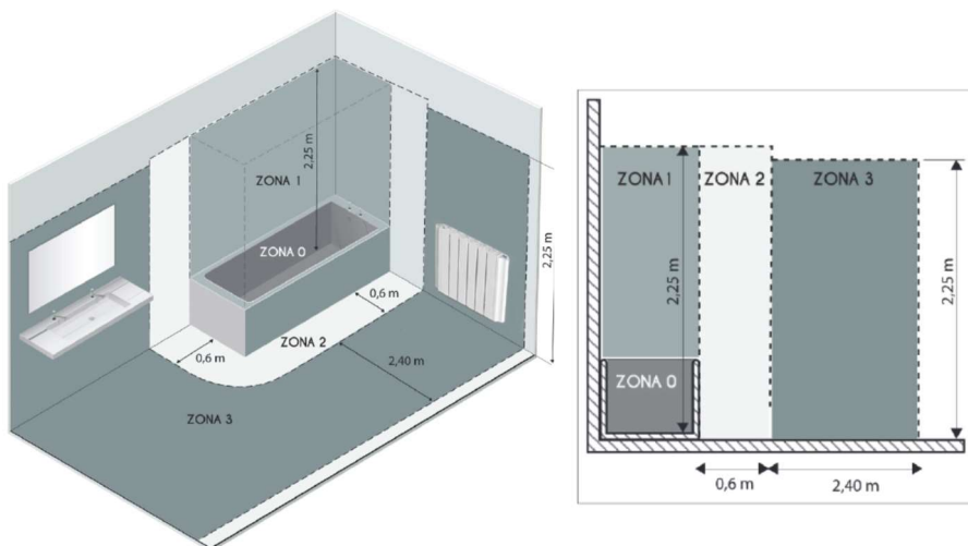
Volume 1: Aparelhos da Muito Baixa Tensão de Segurança (MBTS). Volume 2: Aparelhos elétricos Classe II – IP X4 Volume 3: Aparelhos elétricos protegidos por meio de um dispositivo diferencial de corrente diferencial estipulada I_{\Delta n} não superior a 30 mA. Fig.2
